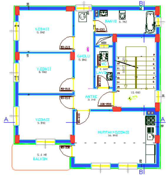
ZEMİN KAT PLANI Ö:1/50
