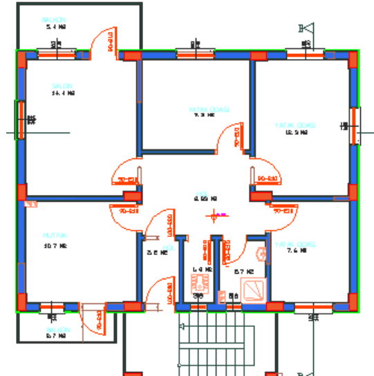
ZEMİN KAT PLANI Ö:1/50
