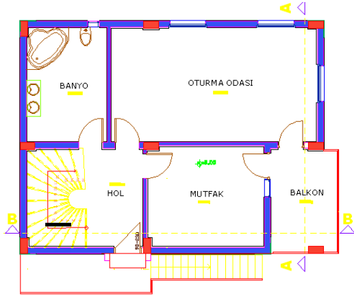
ZEMİN KAT PLANI Ö:1/50
