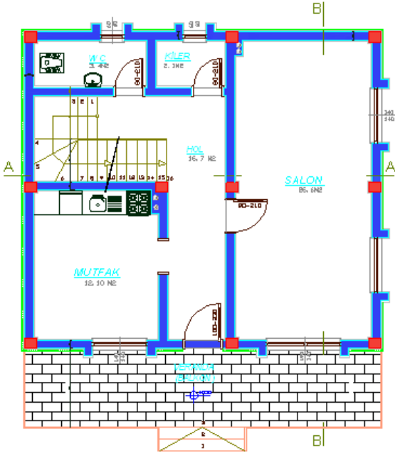
ZEMİN KAT PLANI Ö:1/50
